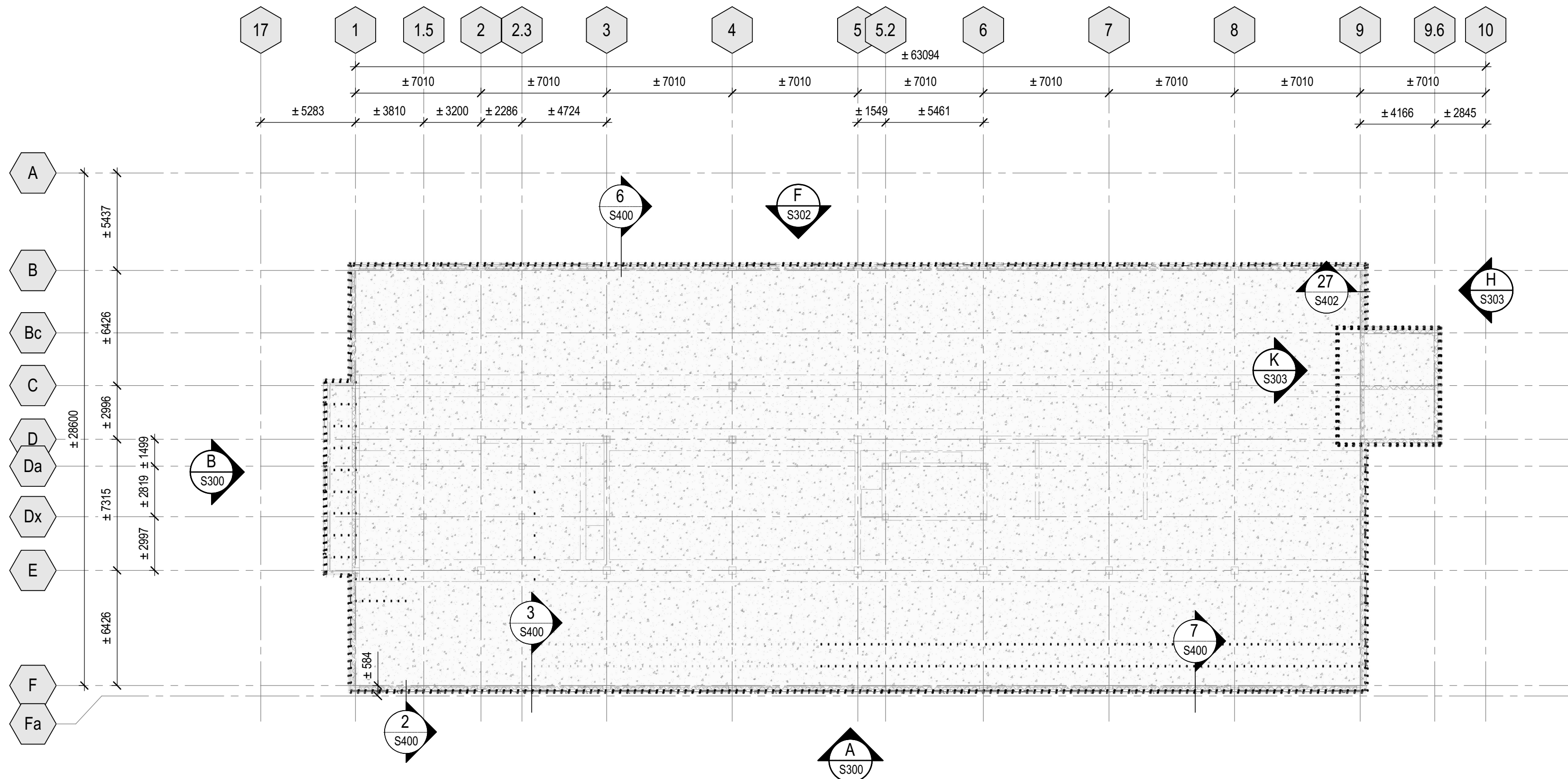
VUE EN PLAN NIVEAU 500 - CONSTRUCTION
