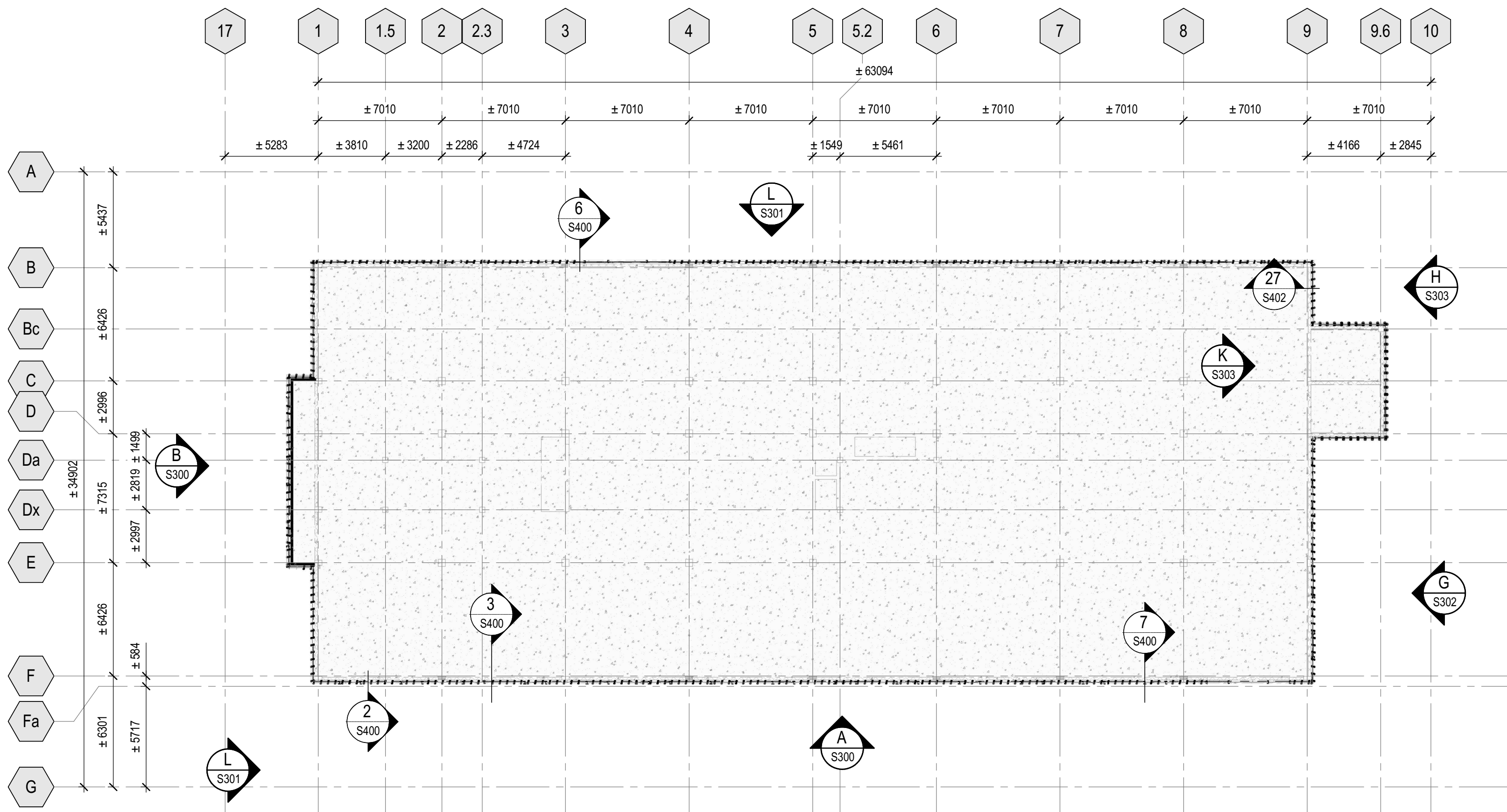
VUE EN PLAN NIVEAU 400 - CONSTRUCTION
