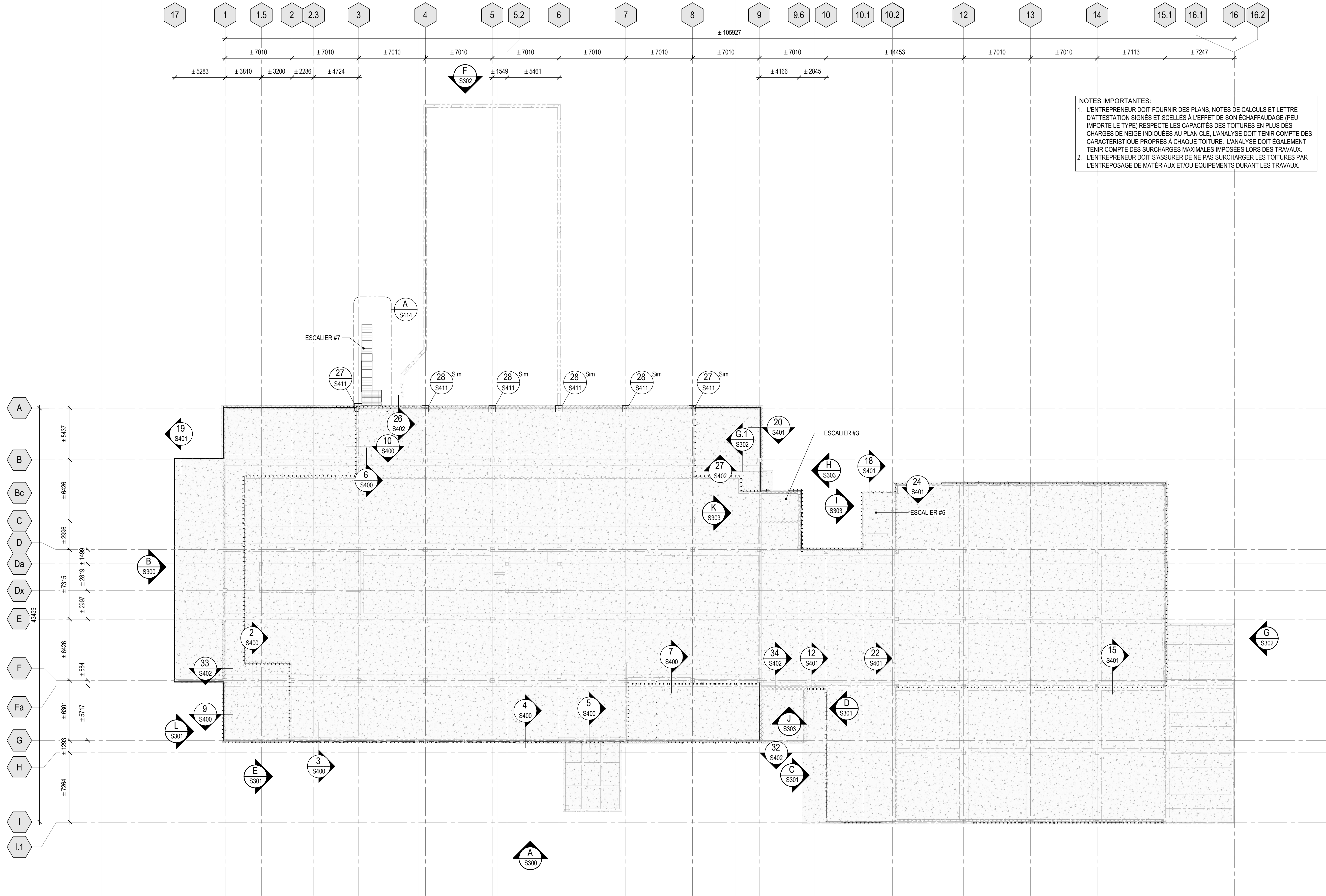
VUE EN PLAN NIVEAU 100 - CONSTRUCTION
