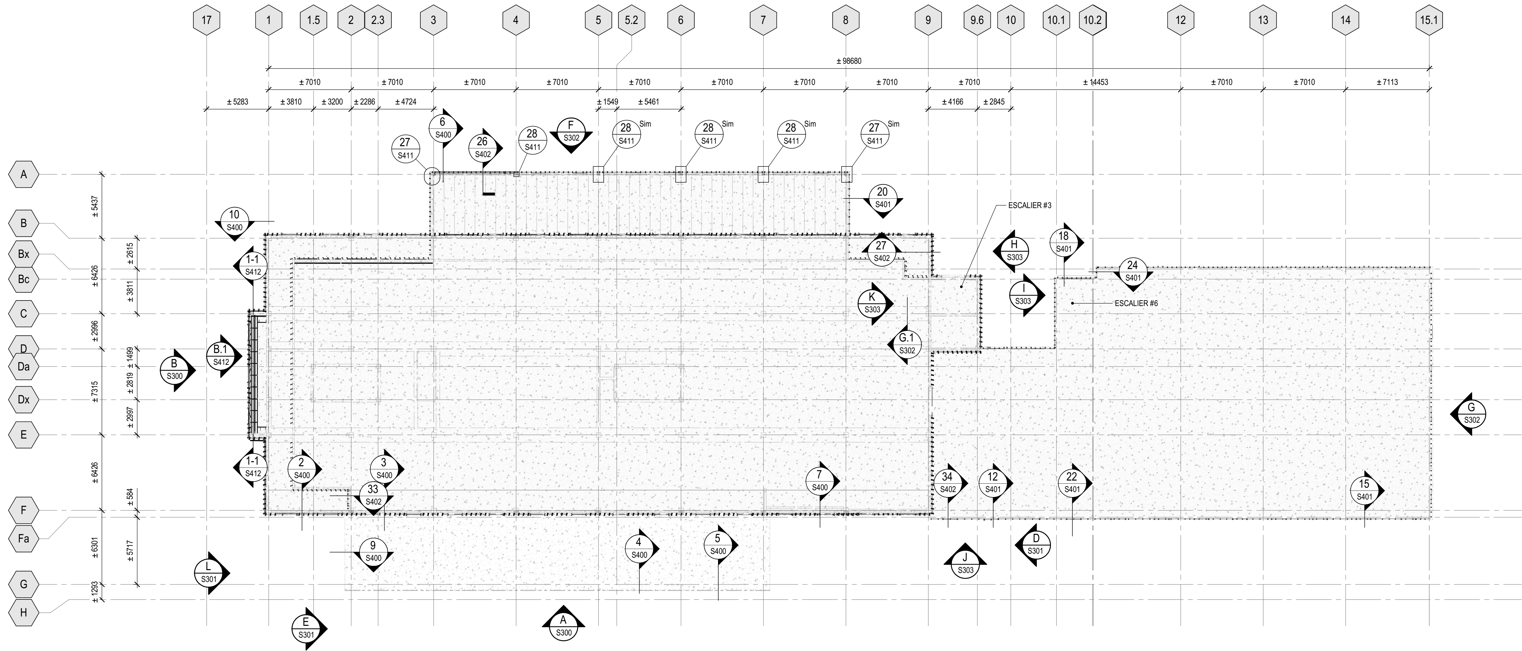
VUE EN PLAN NIVEAU 200 - CONSTRUCTION
